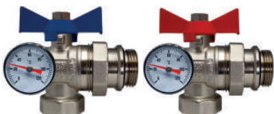
Zawór z srubunkiem Nickel KHT 1' katowy z uszczelką + termometr (niebieski, czerwony)
