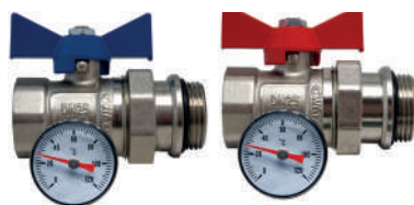
Zawór z srubunkiem Nickel KHT 1' prosty z uszczelką + termometr (niebieski, czerwony)
