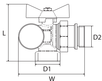
Кран американка Brass KHT 1" кутовий з прокладкою + термометр blue/ red VAK-B-IP-B
